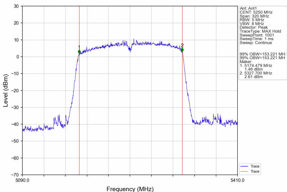
802.11ax(HEW160)_MCH_5250MHz_2xRU996_Left_Ant1_NTNV
