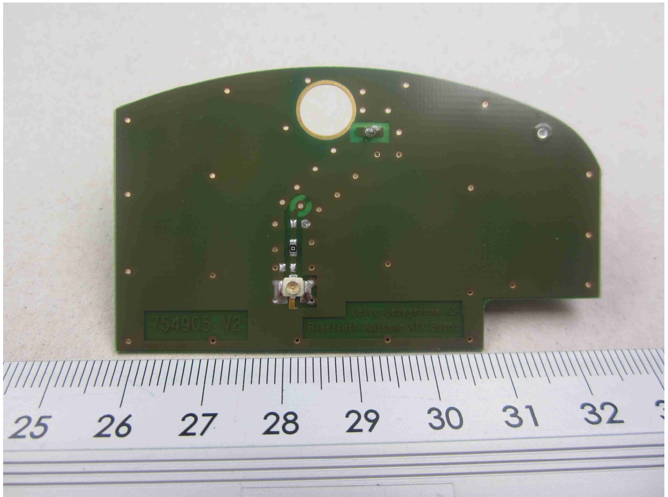
130857_18.JPG: BTAB-2450 Antenna bottom view
