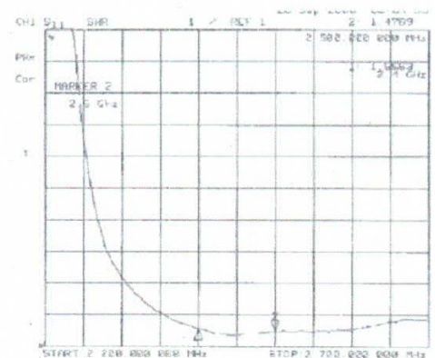
VSWR
