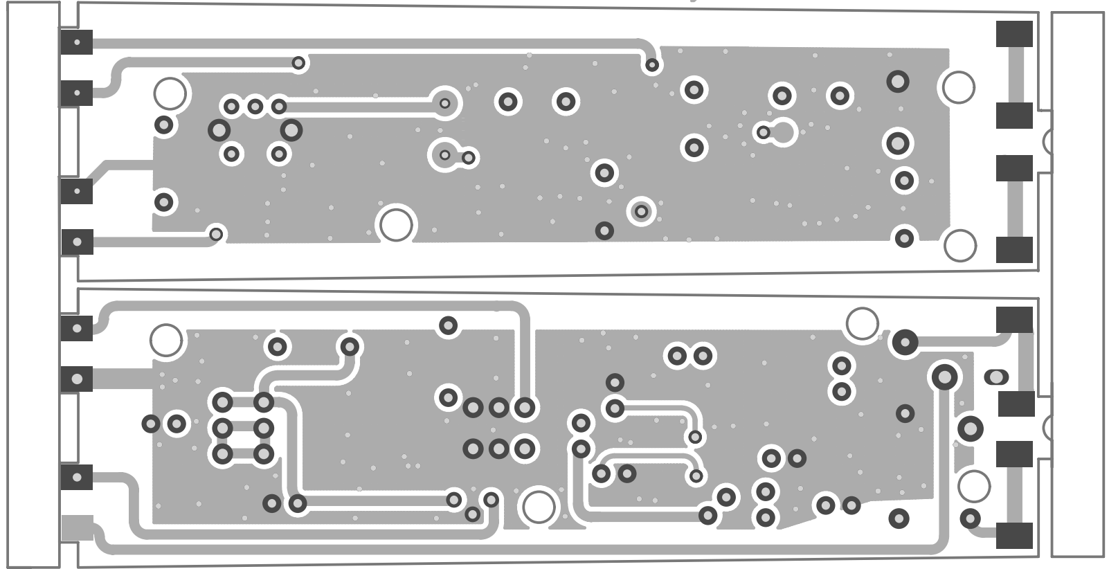
HT-V20 Transmitter Bottom Layer
