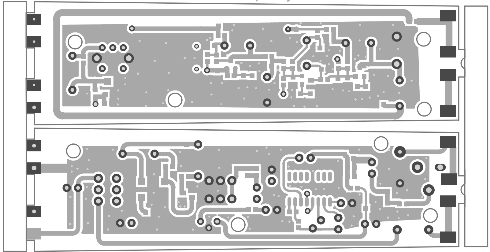
HT-V20 Transmitter Top Layer
