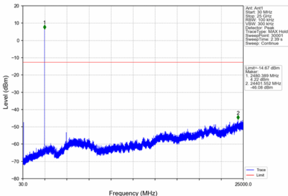
GFSK_DH5_HOPP_Ant1_NTNV
