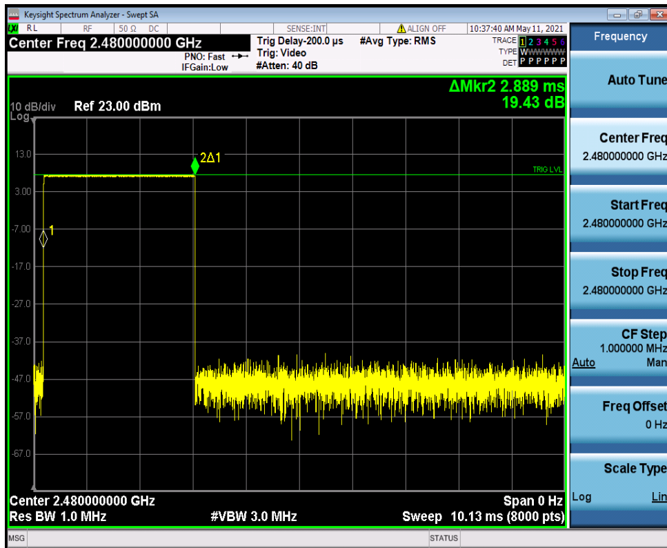
DH5_Ant1_Hop_2480
