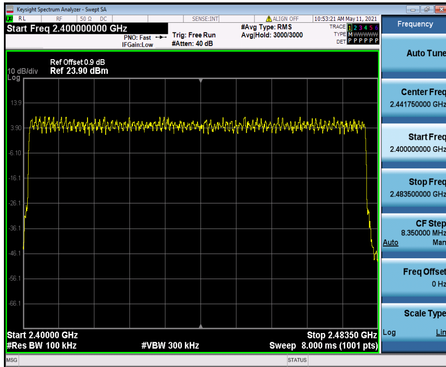
3DH5_Ant1_Hop
