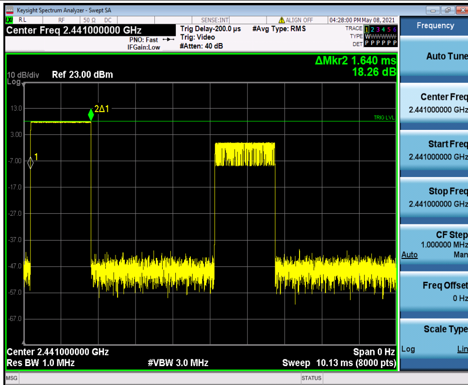
DH3_Ant1_Hop_2441
