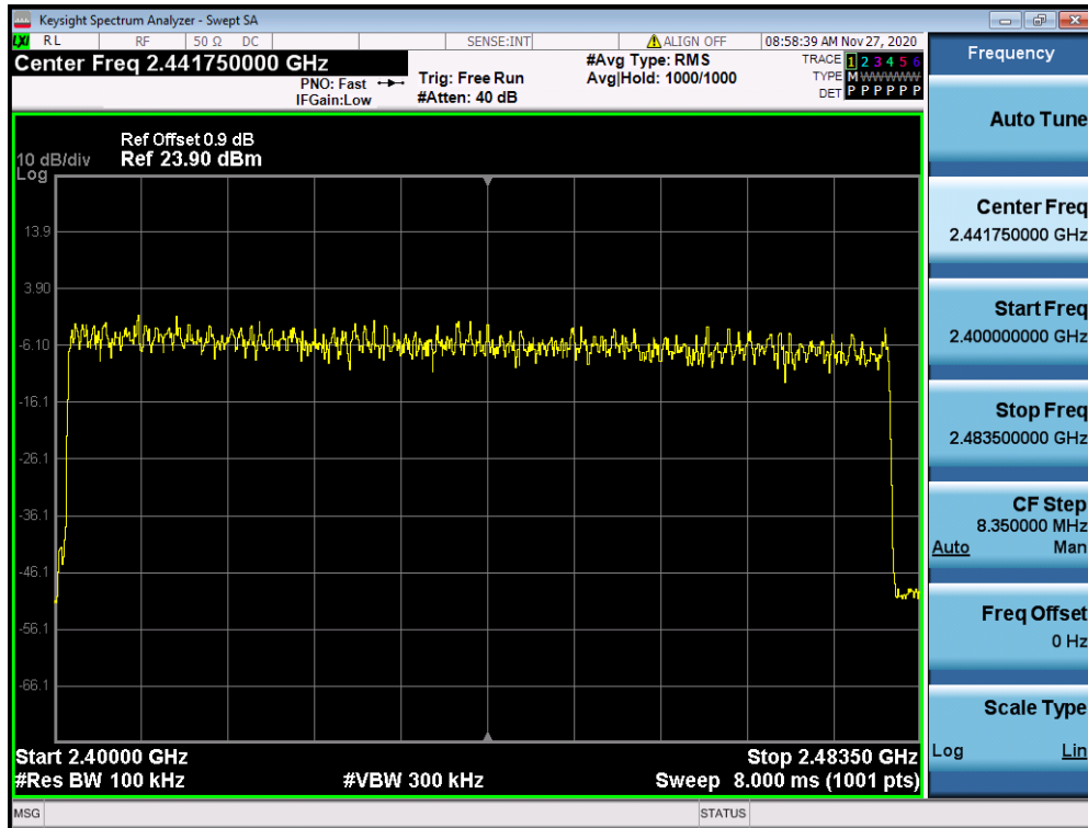
3DH5_Ant1_Hop
