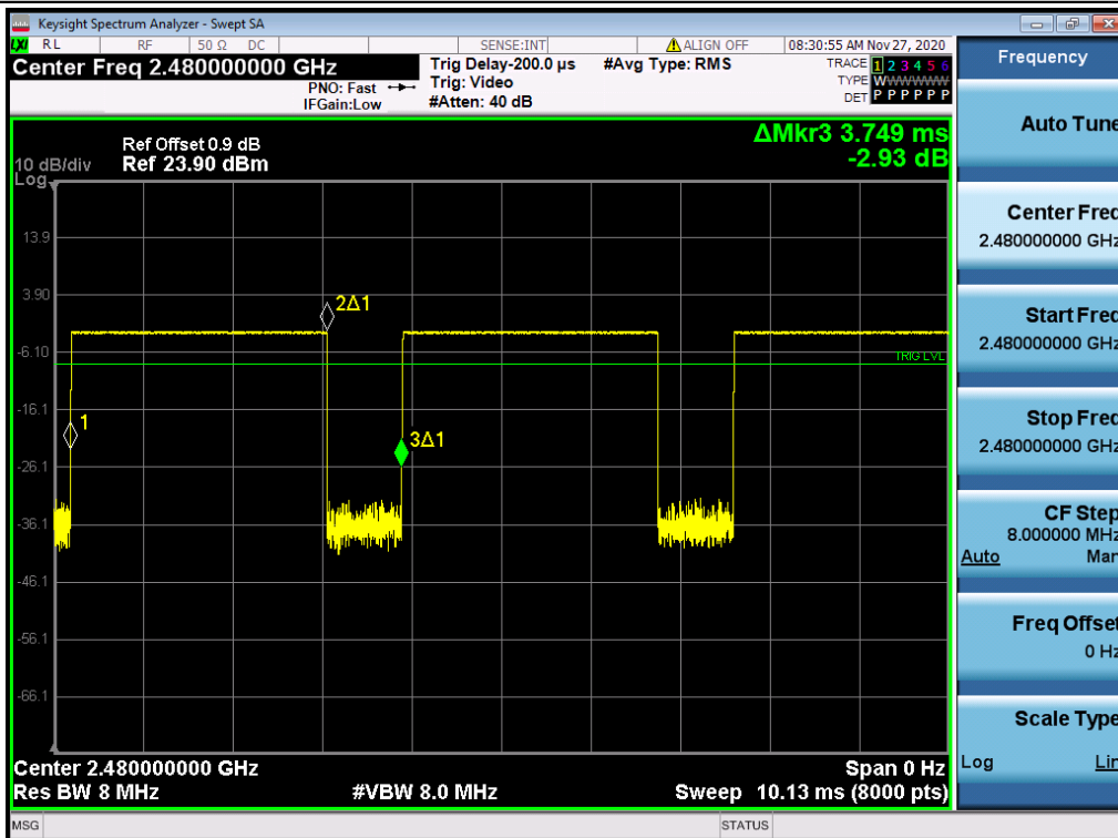
DH5_Ant1_2480
