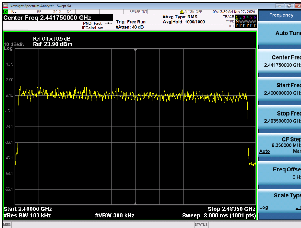
3DH5_Ant1_Hop
