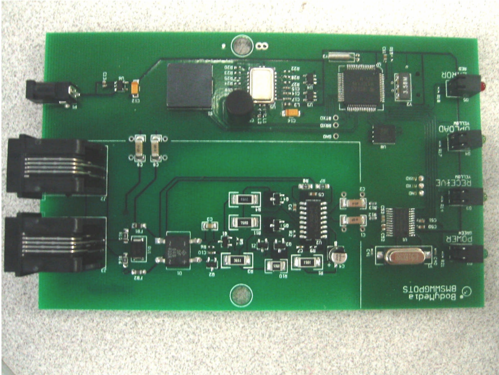
PCB top
