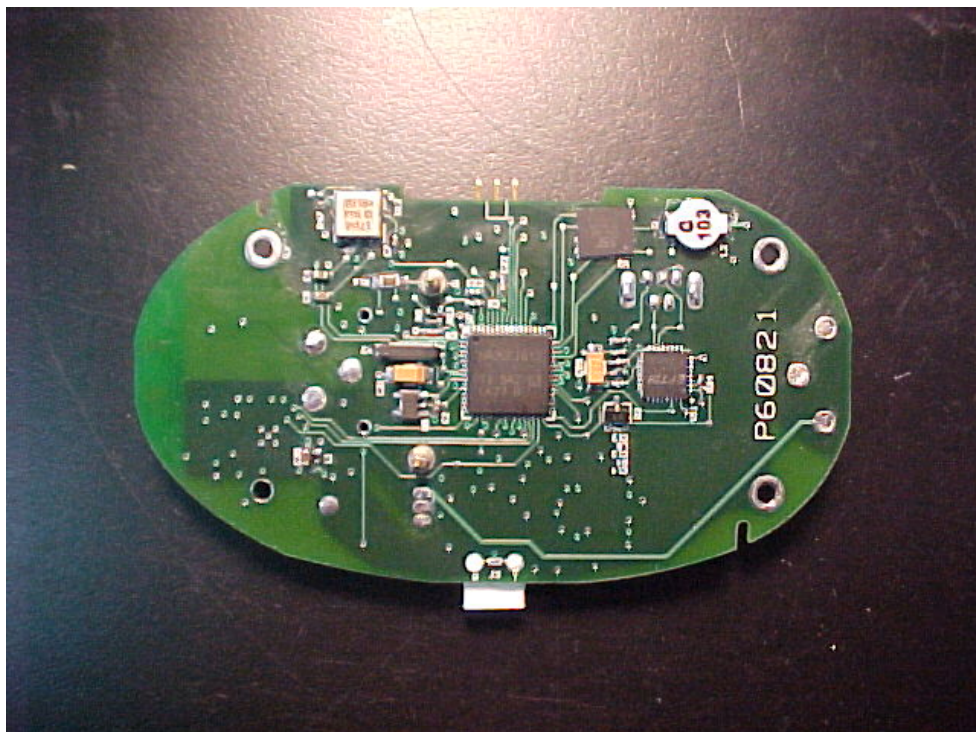
PCB bottom
