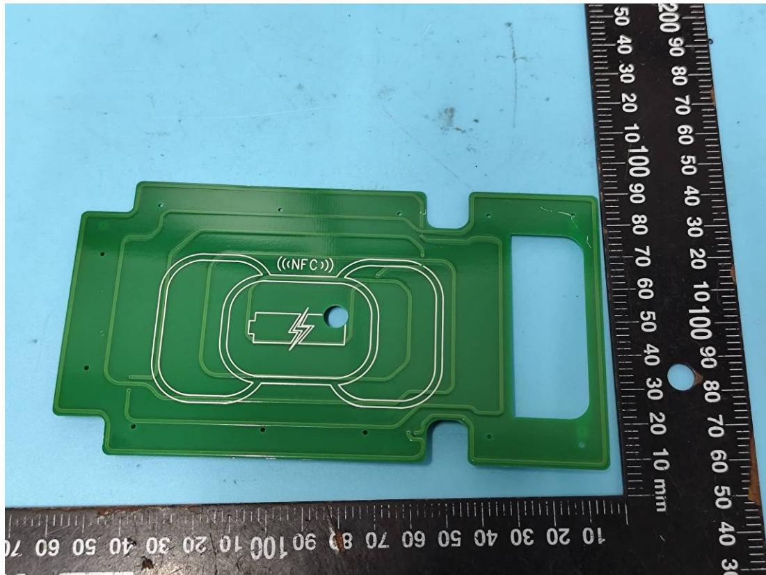
NFC ANT
