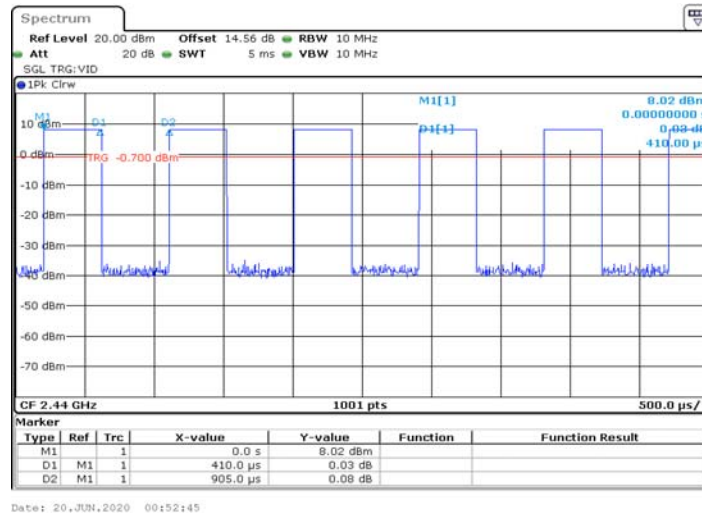
LE 2M_Ant1_2440
