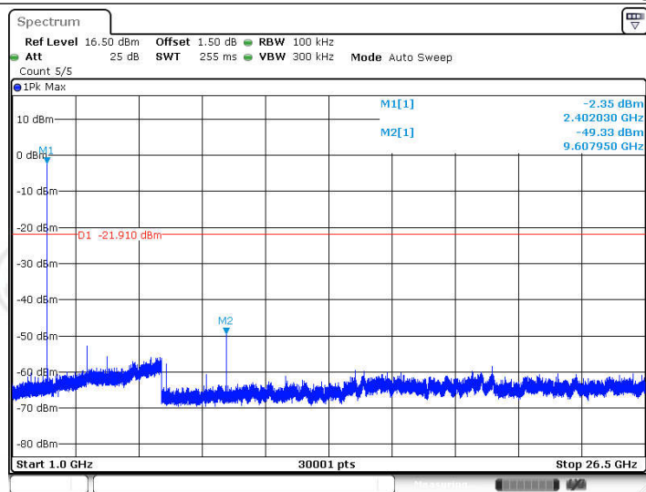
DH5_Ant1_2402_1000~26500
