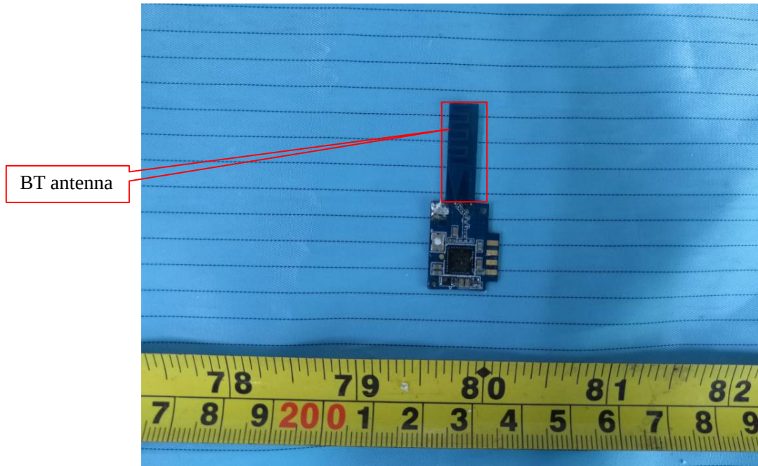
EUT –BT Module Top View
