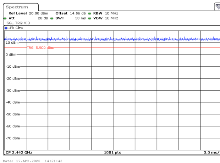
11N20_Ant1_2442
