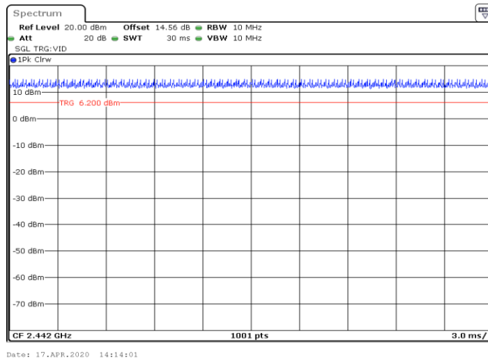
11N20_Ant1_2442
