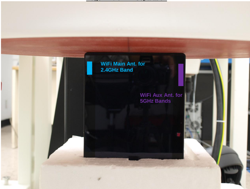
Edge 3 w/ 0 mm Separation
