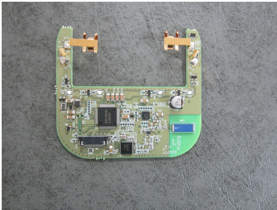
BOT PCB RFMT-3
