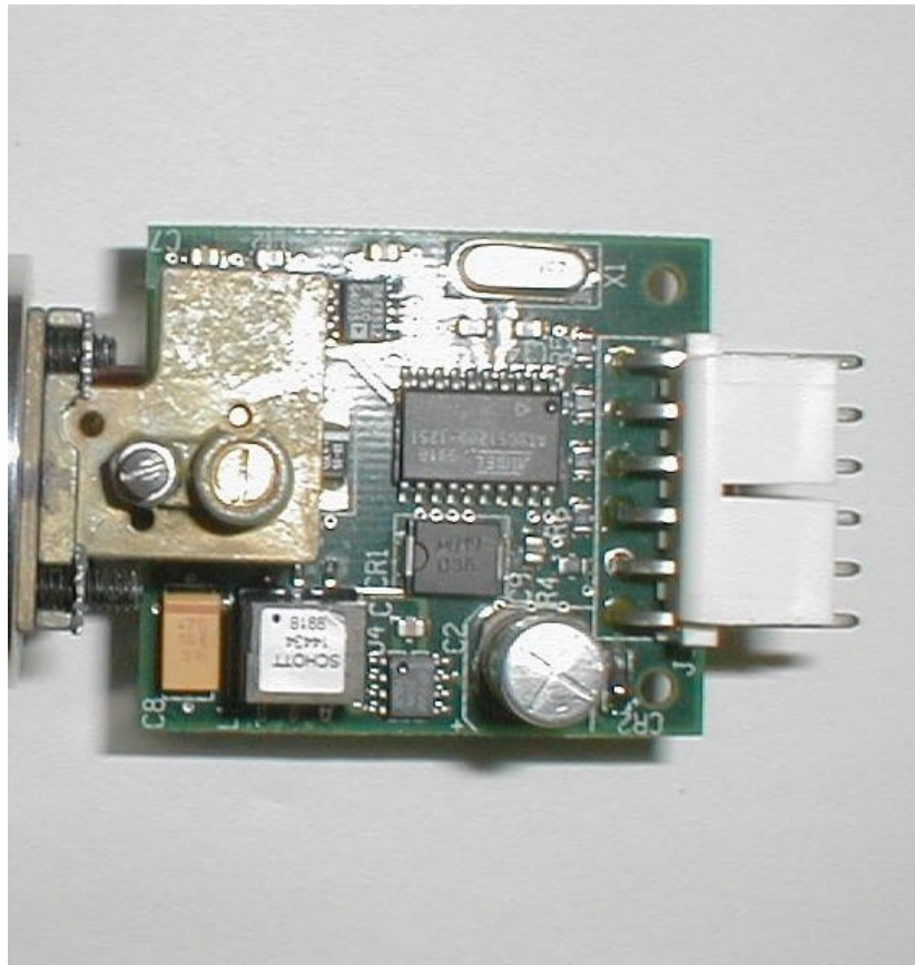
PCB Bottom
