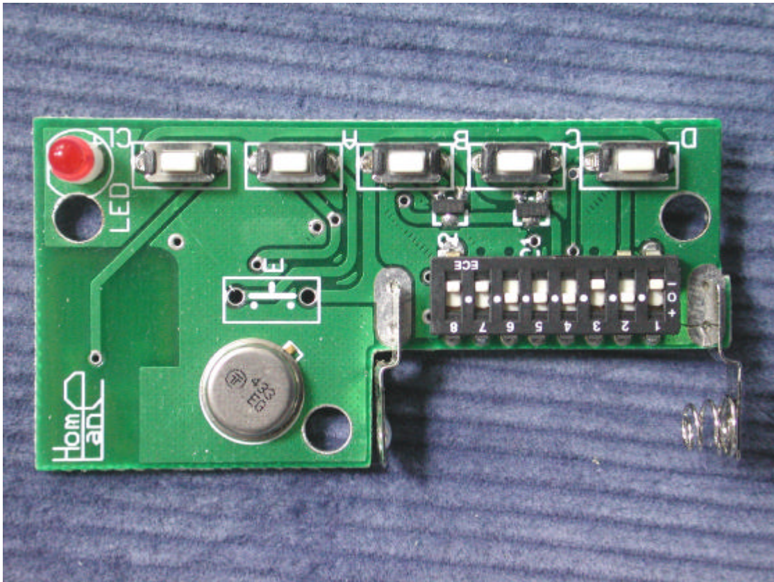
(6) EUT Photo
