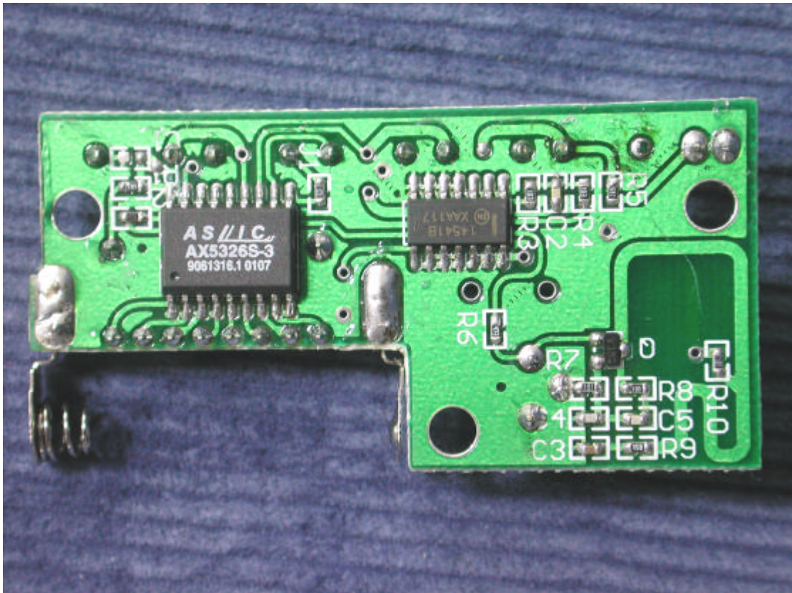
(6) EUT Photo
