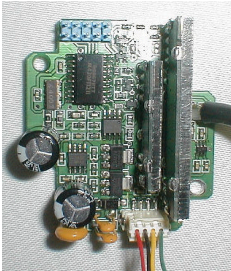
PCB Bottom
