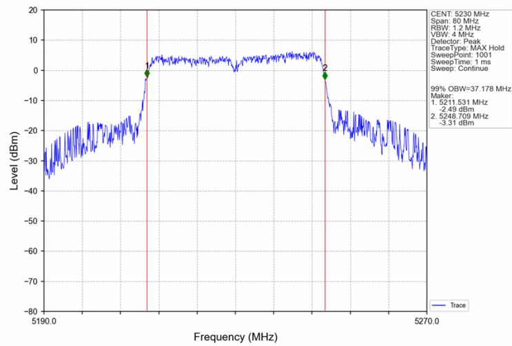
802.11n(HT40)_HCH_5230MHz_Ant2_NTNV
