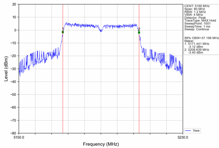
802.11n(HT40) LCH_5190MHz_Ant2_NTNV
