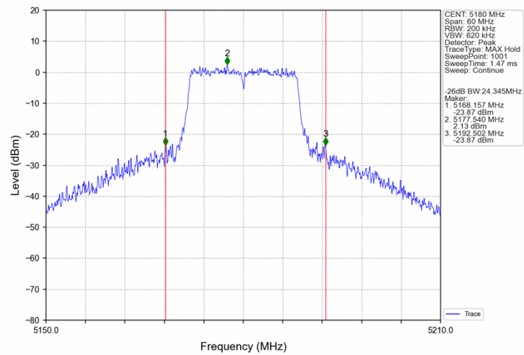
802.11a_LCH_5180MHz_Ant2_NTNV
