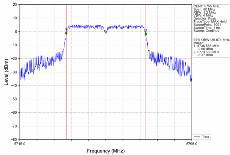
802.11n(HT40) LCH_5755MHz_Ant2_NTNV
