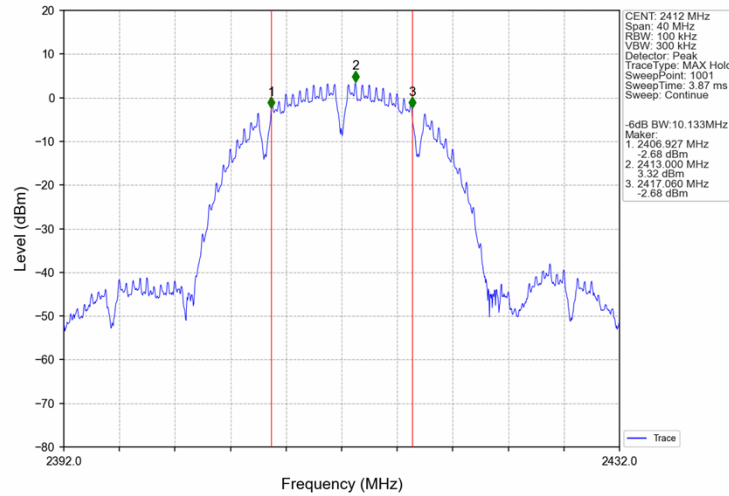
802.11b_LCH_2412MHz_Ant2 (SISO)_NTNV
