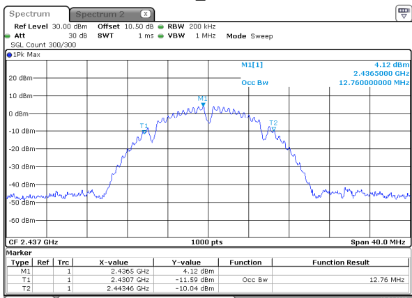
802.11b_2437MHz
