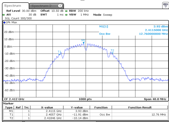
802.11b_2412MHz
