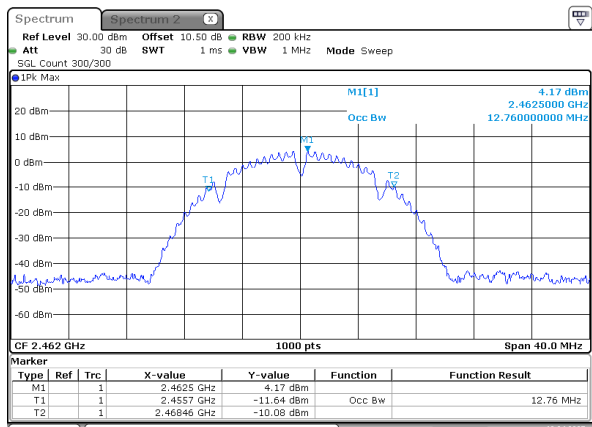
802.11b_2462MHz
