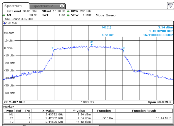
802.11g_2437MHz
