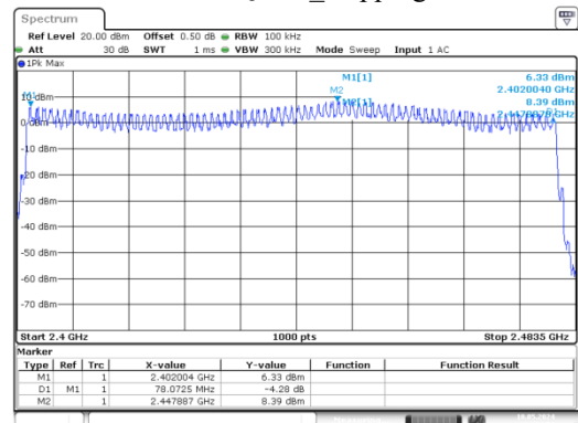
\pi/4 -DQPSK_Hopping
