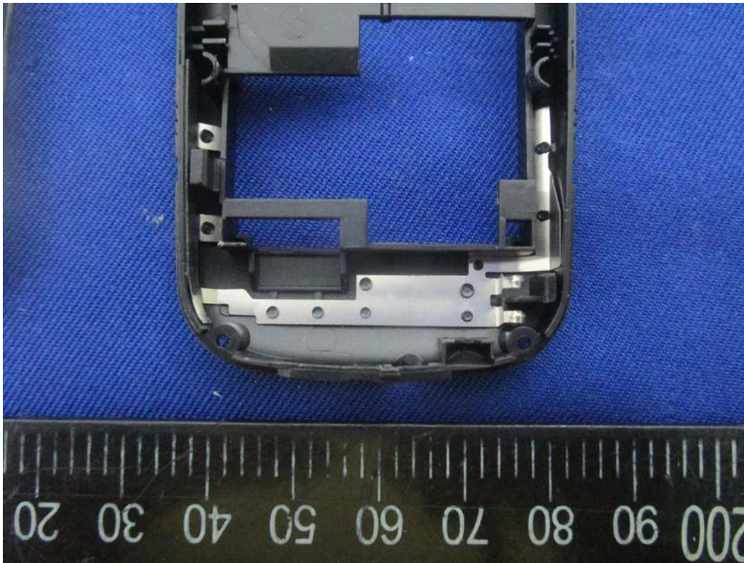
GSM Antenna
