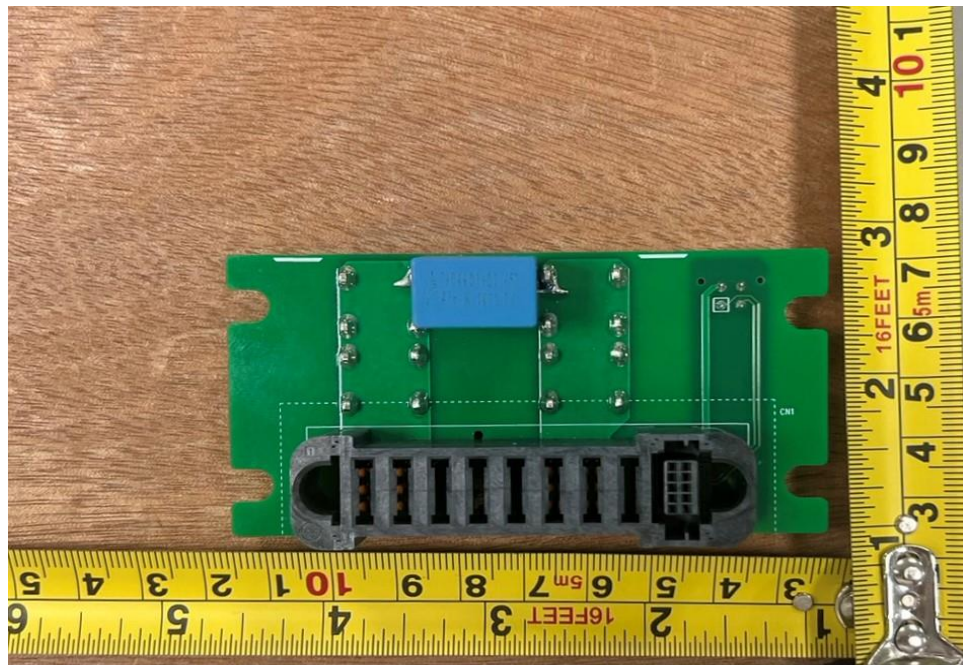
EUT Photo (152)
