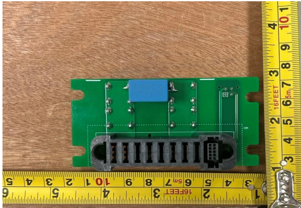
EUT Photo (132)
