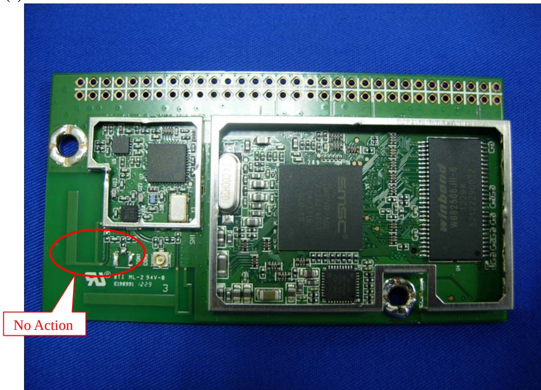
(4) EUT Photo
