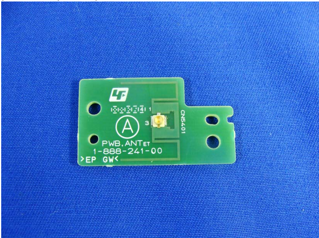
(10) EUT Photo_ (Antenna 1)
