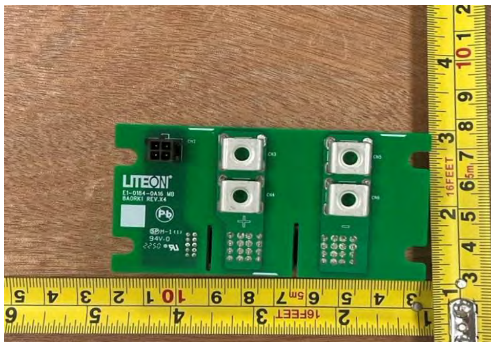
EUT Photo (130)
