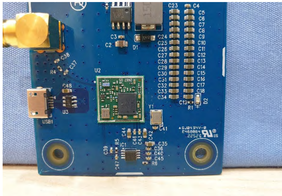
EUT Photo (4)
