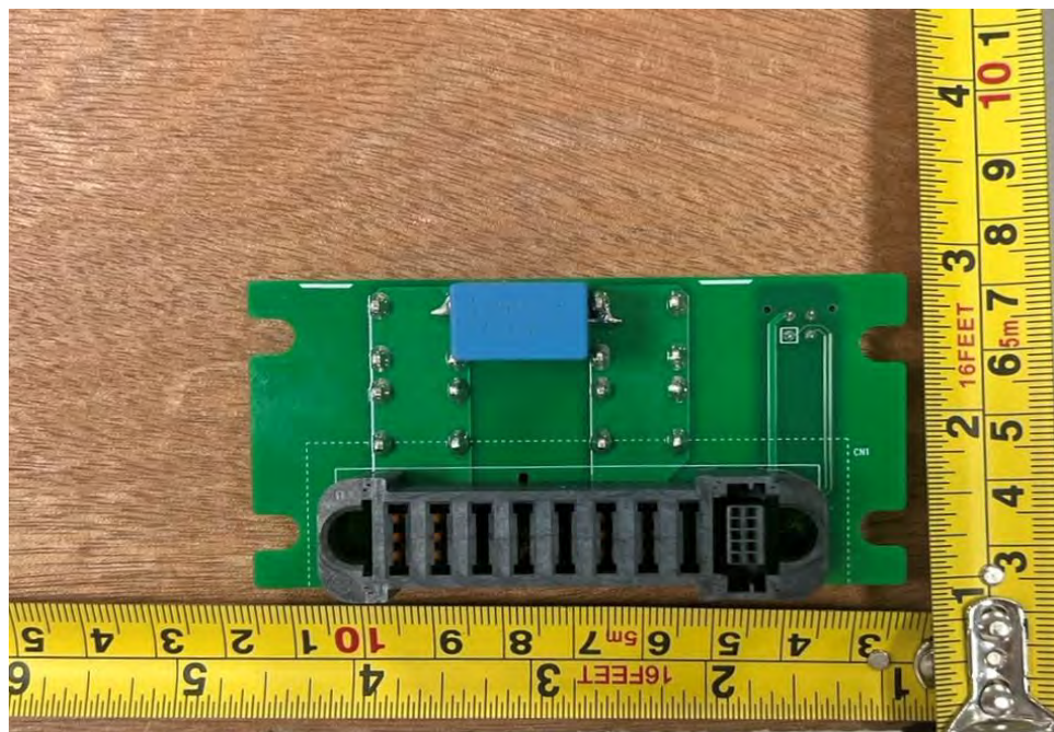
EUT Photo (152)
