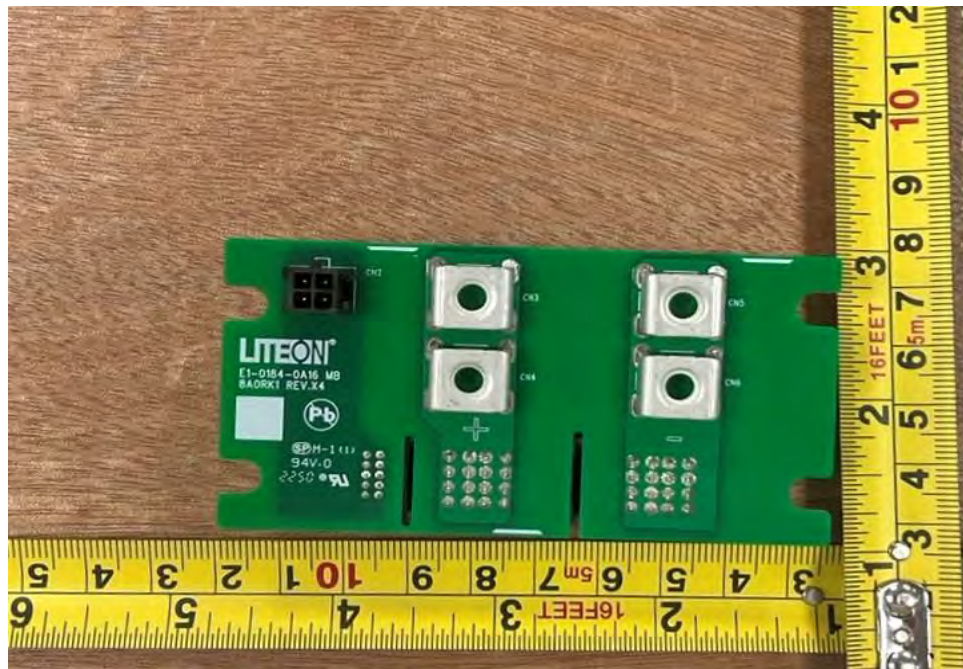
EUT Photo (156)
