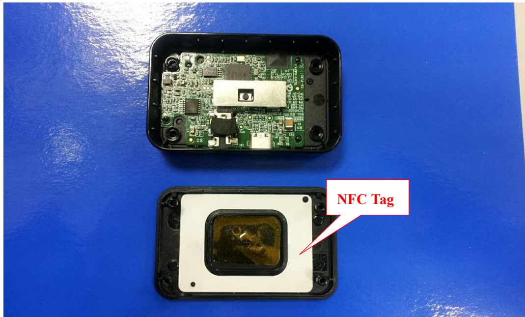
(5) EUT Photo
