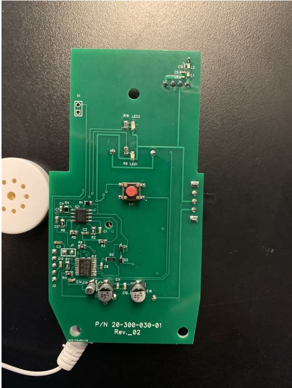
PCB Top
