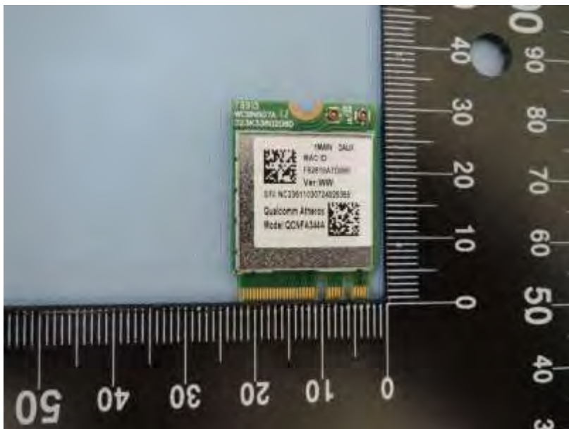
Fig.10 Back view_2
