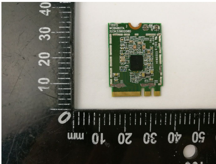
RF MODULE (QCNFA344A)-2
