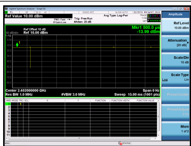
2DH5 2402MHz
