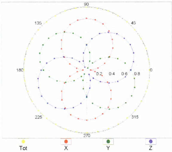
f=450 MHz,TEM
