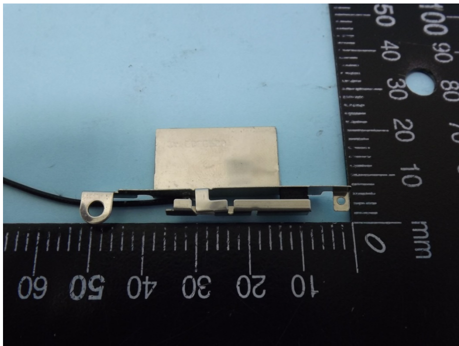
PIFA Antenna
