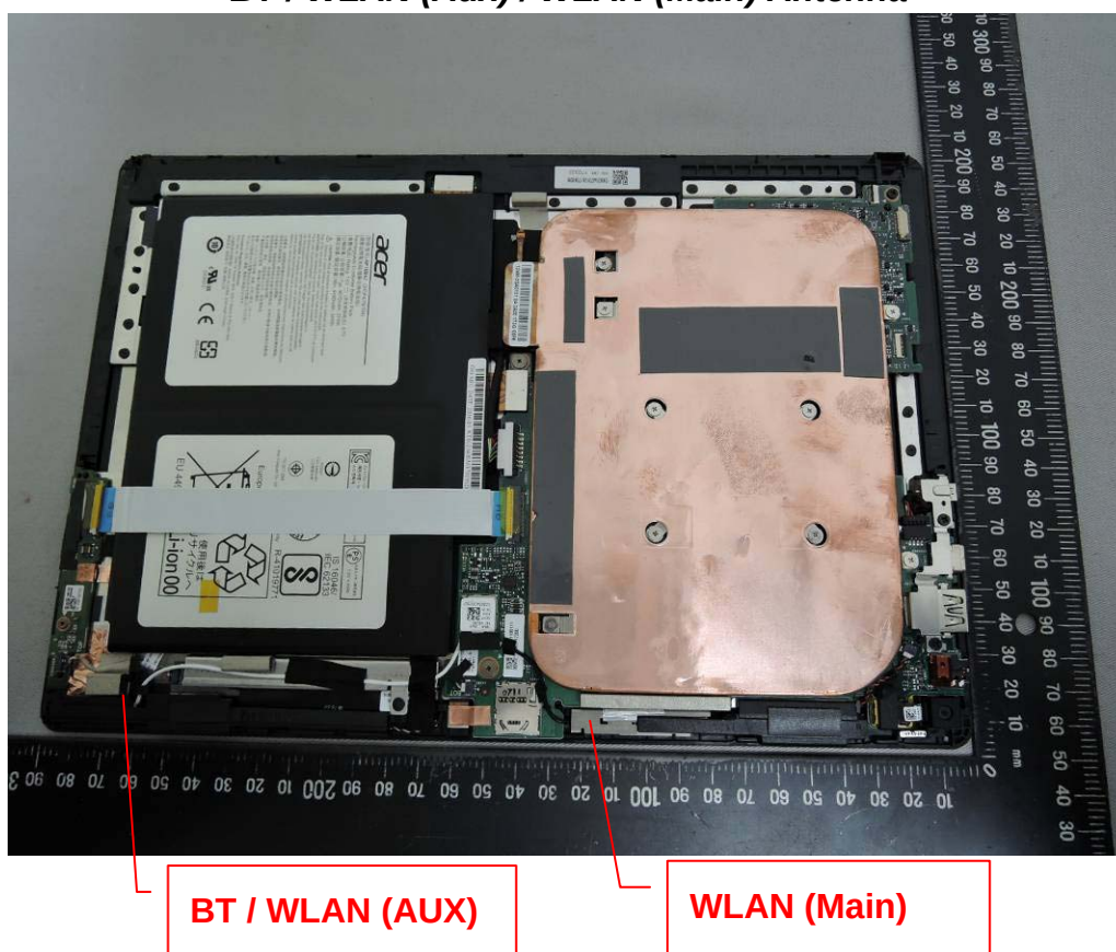
BT / WLAN (Aux) / WLAN (Main) Antenna
