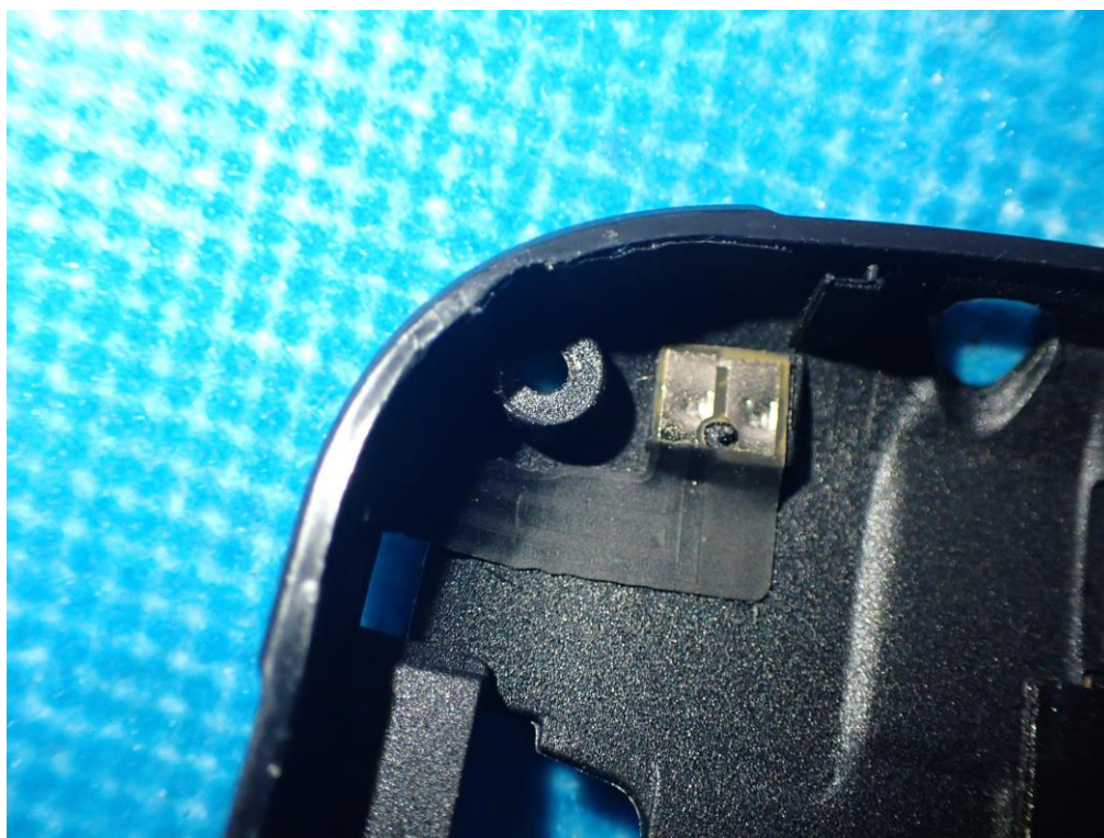
BT&WIFI&GPS ANTENNA
