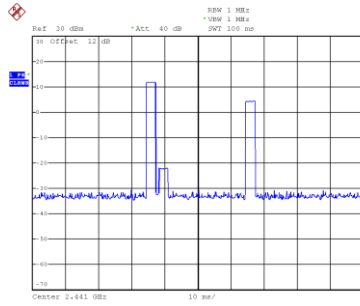
CH39- DH5
