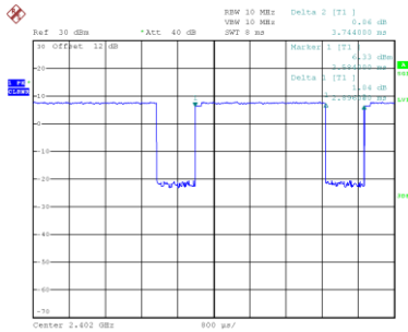
CH00-2DH5
