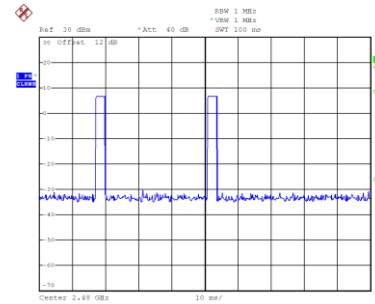
CH78-2DH5
