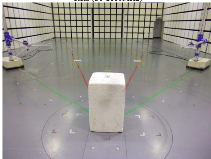
Rear (30-1000MHz)
