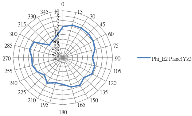
Phi_E2 Plane(YZ)
