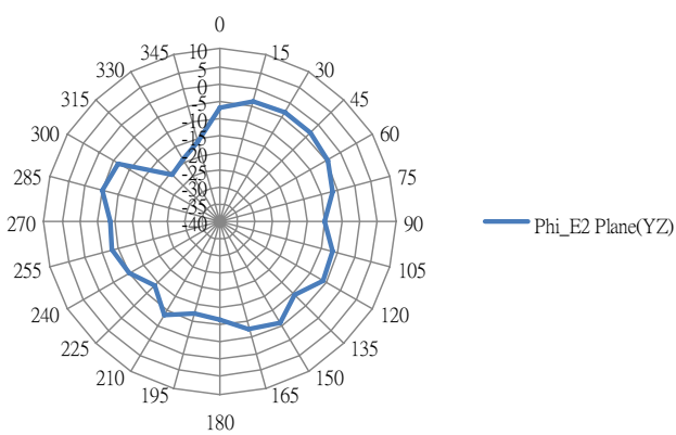
Phi_E2 Plane(YZ)
