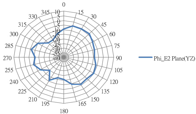
Phi_E2 Plane(YZ)
