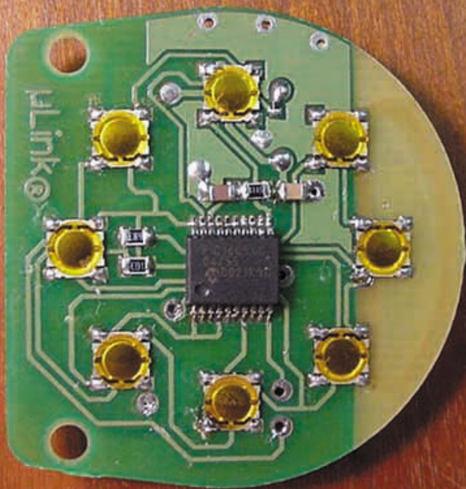
418MHz circuit top
