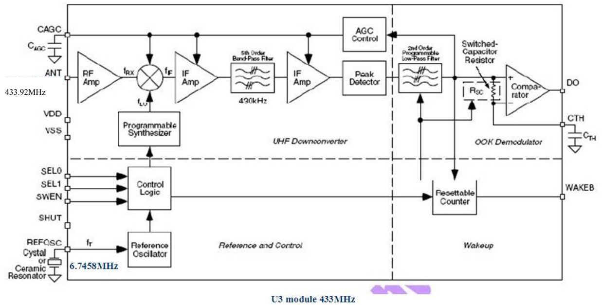
U3 433MHz module Block
