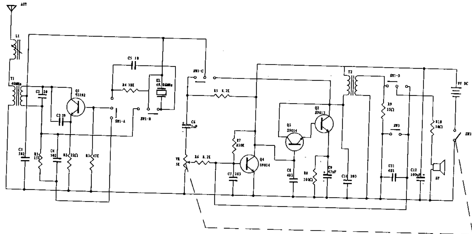
對講機線路圖
