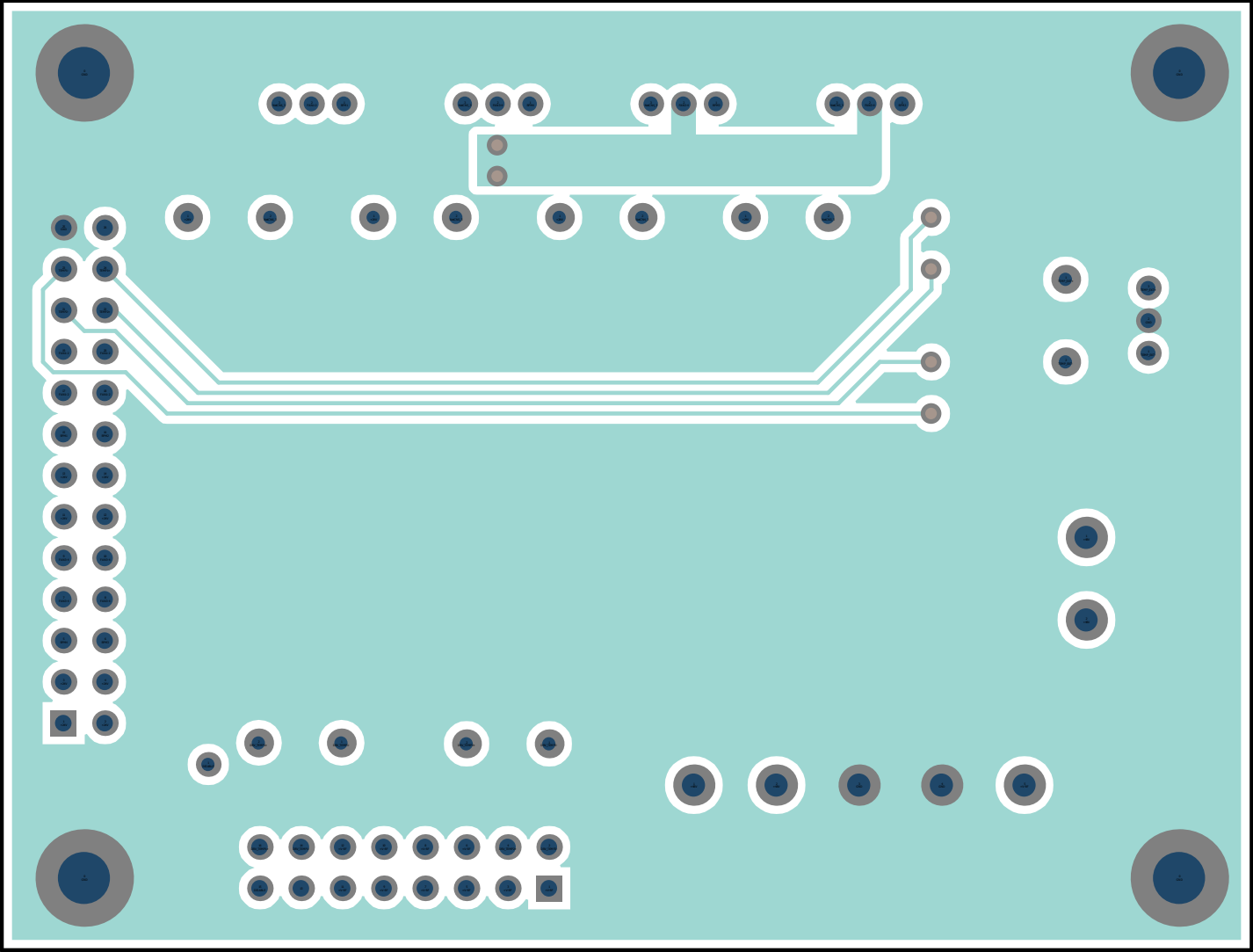
Bottom Layer Bottom Overlay
