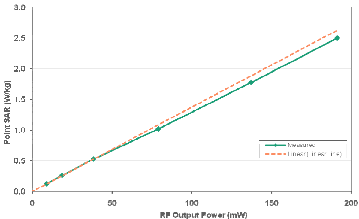
5 MHz, QPSK
