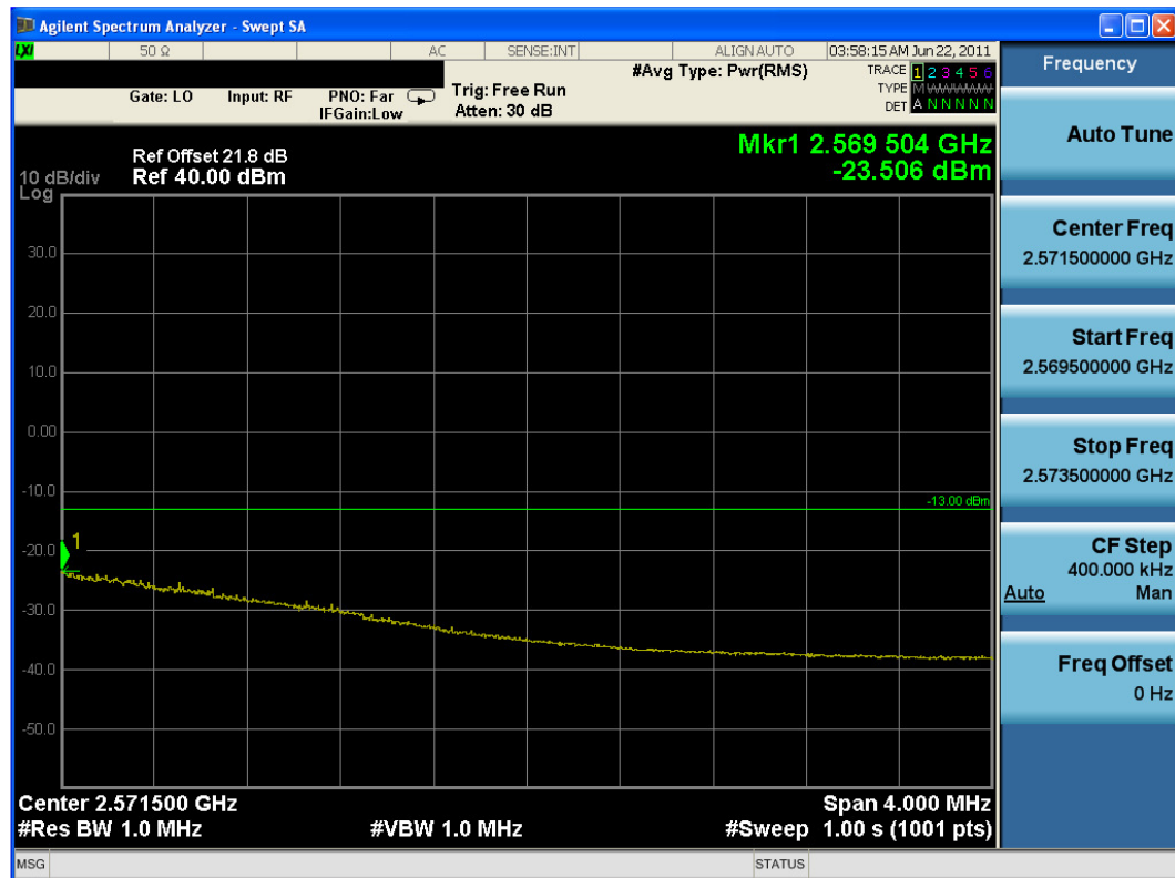
Plot 7-6. Hi 4MHz Plot (TD-CDMA - QPSK) Antenna Port 1
